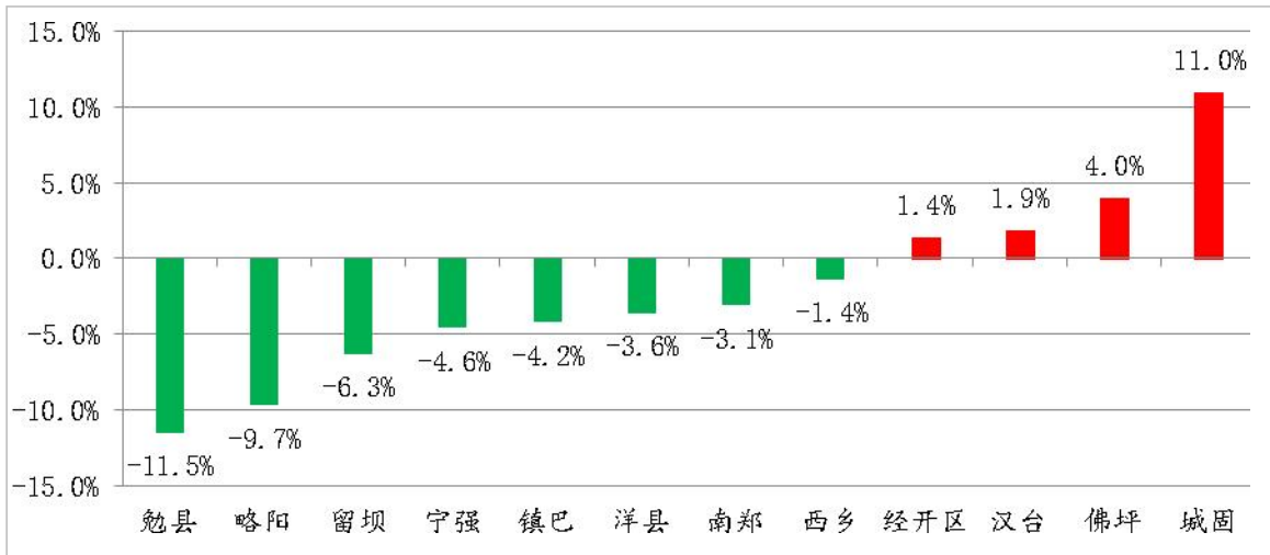
图4 2022年6月各县区环境空气质量综合指数同比变化情况
