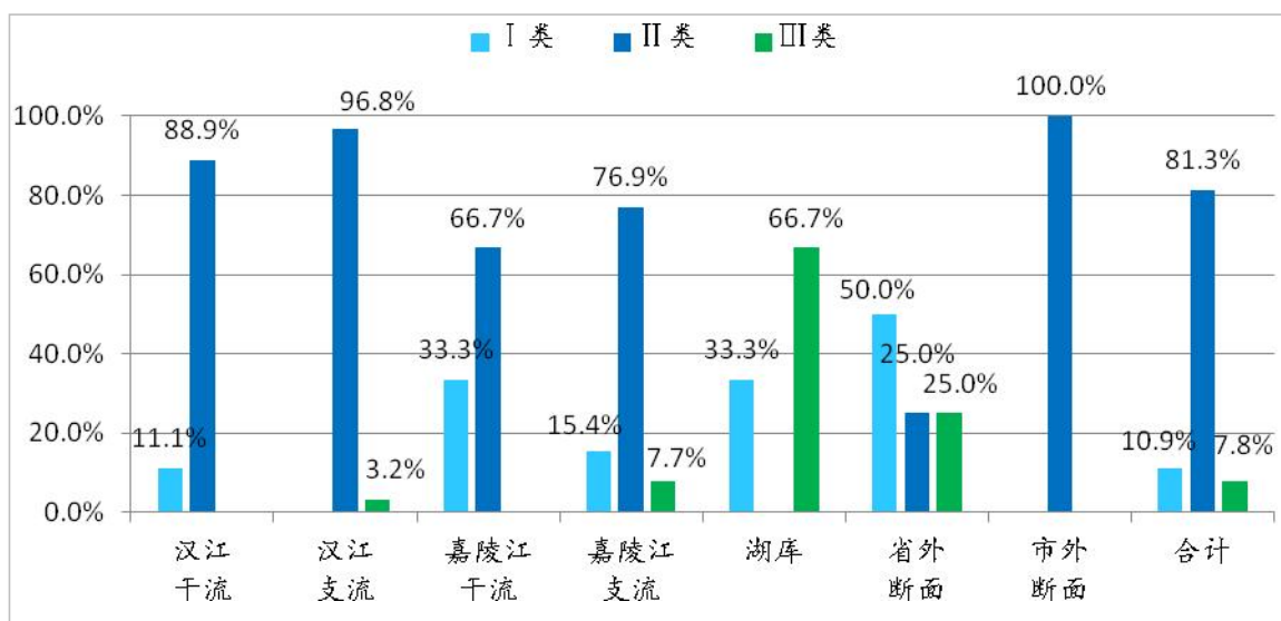
图 9 2022 年 6 月全市地表水断面水质类别比例图
