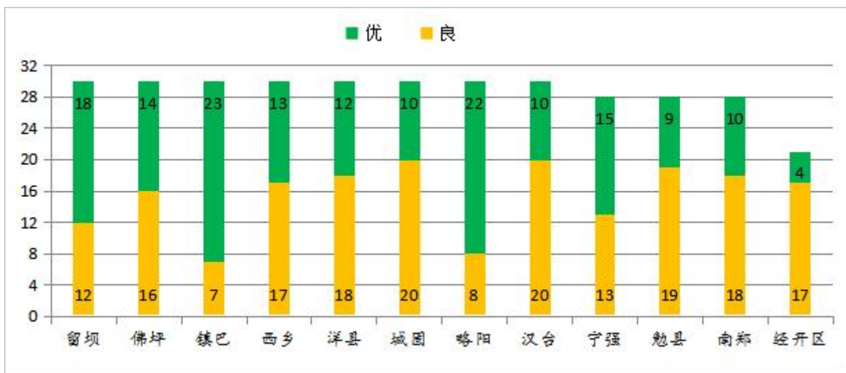
图1 2022年6月各县区环境空气质量优良天数图(单位:天)
