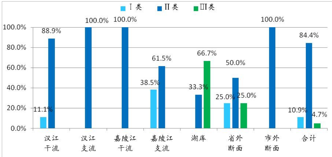
图 10 2022 年 1~6 月全市地表水断面水质类别比例图
