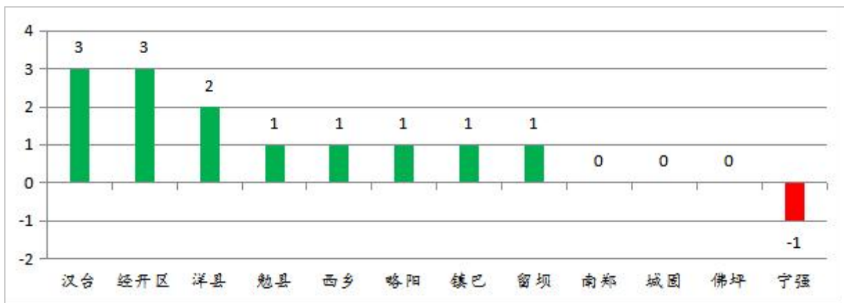
图2 2022年6月各县区环境空气质量优良天数同比变化情况(单位:天)
