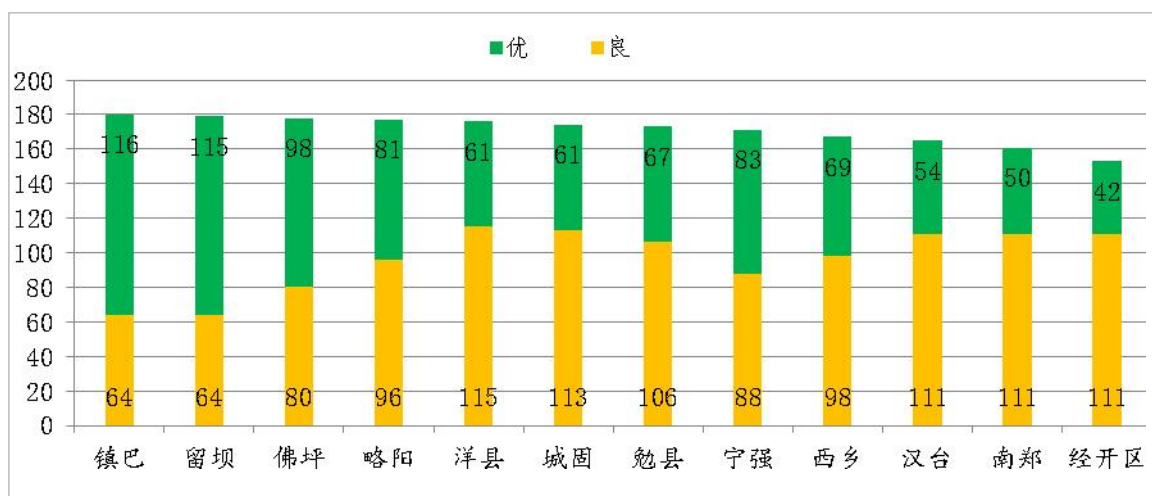
图 5 2022 年 1~6 月县区环境空气质量优良天数（单位：天）
