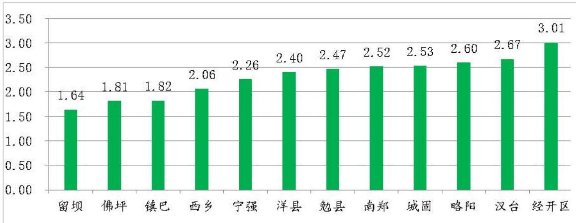
图3 2022年6月各县区环境空气质量综合指数
