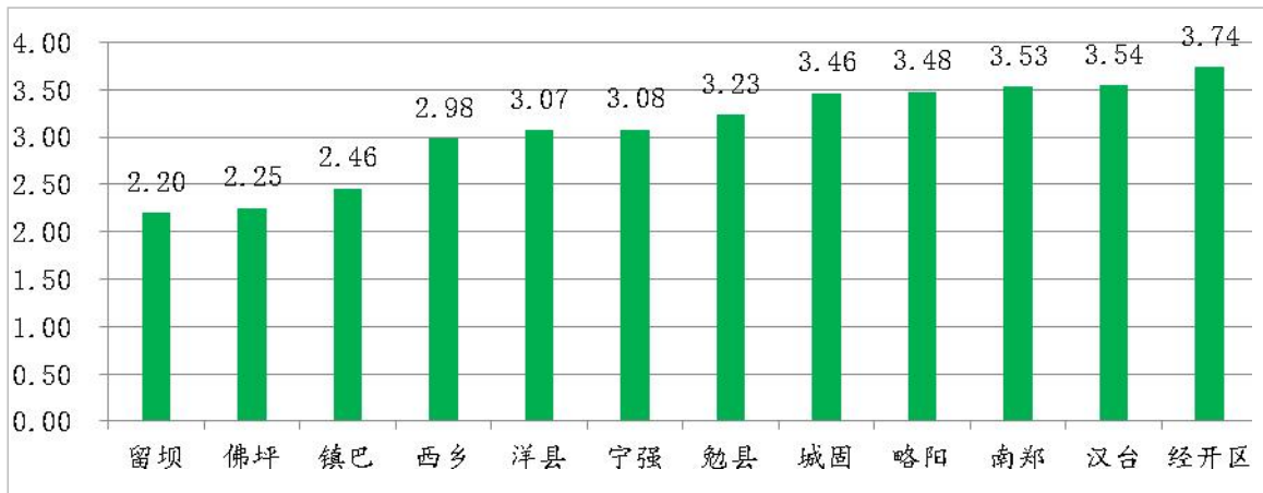
图7 2022年1~6月县区环境空气质量综合指数
