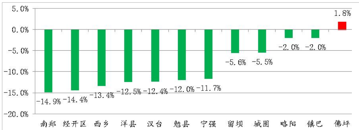
图8 2022年1~6月县区环境空气质量综合指数同比变化情况
