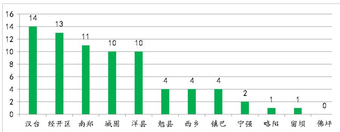
图6 2022年1~6月县区环境空气质量优良天数同比变化情况
